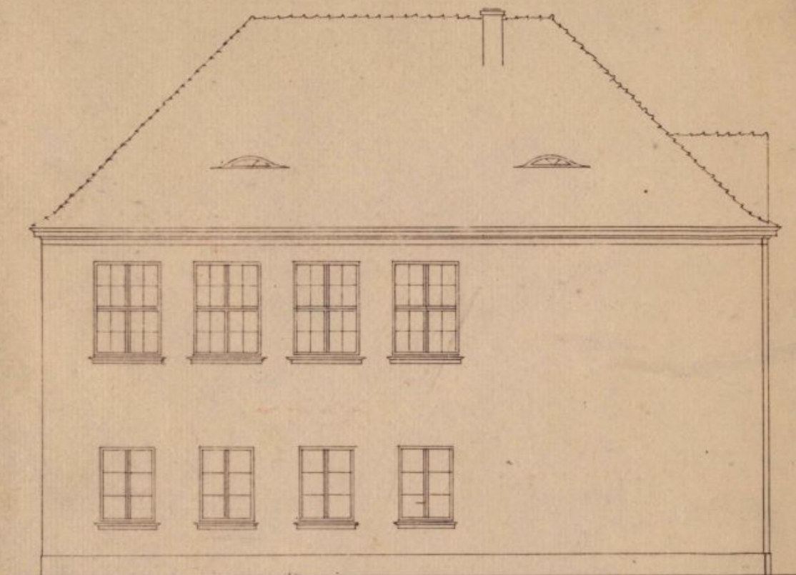
ELEWACJA BOCZNA
