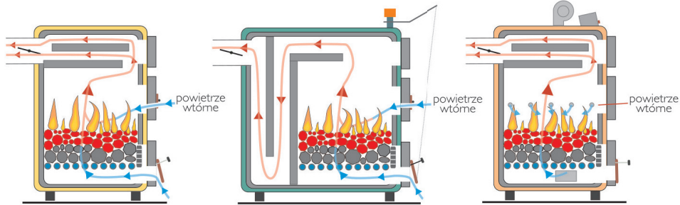
Kocioł z poziomym wymiennikiem
