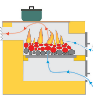
Piec kuchenny
