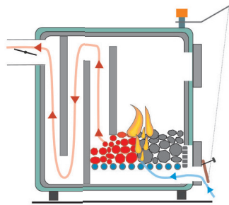
Kocioł górno-dolny
