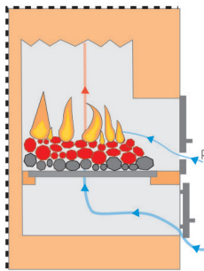
Piec kaflowy
